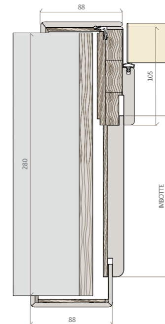
imbotte per spessore muro da 275 a 700 mm compresi jambs for wall thickness 275 to 700 cm chambranles pour épaisseur de mur de 275 à 300 cm inclus tapajuntas para paredes de entre 275 y 300 cm de grosor Verblendungen für Wandstärken von 275 bis einschl. 300 cm накладки для стены толщиной от 275 до 300 см включительно
