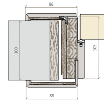
mostrine per spessore muro da 90 a 125 mm compresi jambs for wall thickness 90 to 125 cm chambranles pour épaisseur de mur de 90 à 125 cm inclus tapajuntas para paredes de entre 90 y 125 cm de grosor Verblendungen für Wandstärken von 90 bis einschl. 125 cm накладки для стены толщиной от 90 до 125 см включительно
