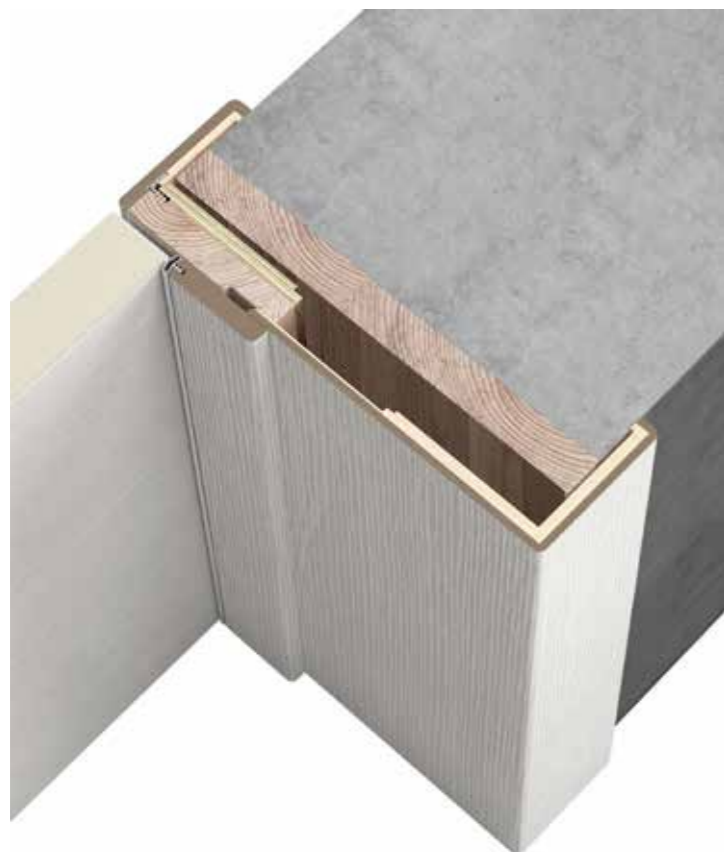
sezione No-Limits con mostrina per spessori muro compresi tra 130 e 270 cm No-Limits jambs with frame for wall thickness of 130 to 270 cm section No-Limits avec chambranle pour épaisseur de mur entre 130 et 270 cm sección No-Limits con tapajuntas para paredes de entre 130 y 270 cm de grosor Querschnitt von No-Limits mit Verblendung für Wandstärken zwischen 130 und 270 cm сечение двери No-Limits с накладкой для стен толщиной от 130 до 270 см
