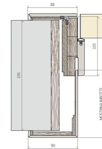
mostrine per spessore muro da 130 a 270 mm compresi jambs for wall thickness 130 to 270 cm chambranles pour épaisseur de mur de 130 à 270 cm inclus tapajuntas para paredes de entre 130 y 270 cm de grosor Verblendungen für Wandstärken von 130 bis einschl. 270 cm накладки для стены толщиной от 130 до 270 см включительно
